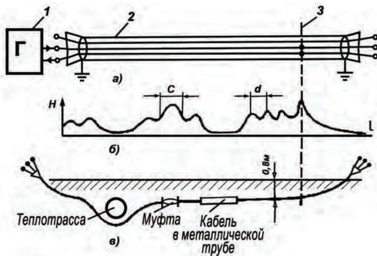
Рис.А.5 КЗ-междупольное
