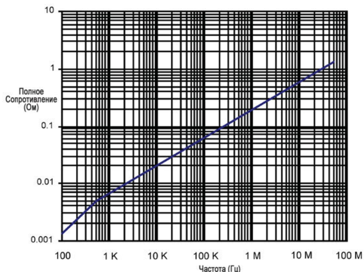
Полное вносимое сопротивление при частоте
