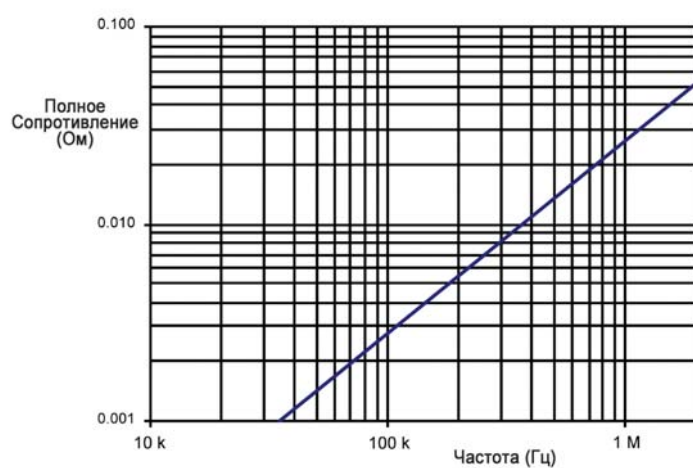
Полное вносимое сопротивление при частоте
