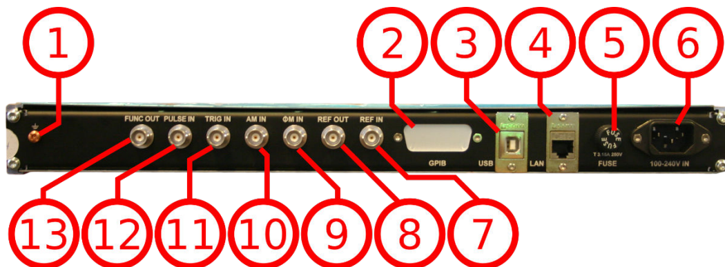
Рис.7:ВидзаднейпанелиAPSIN 1URM
