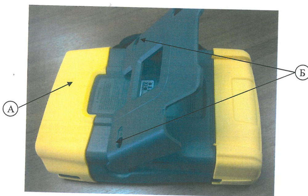
Рисунок 1 - Общий вид осциллографов Fluke 190-104, 190-204
