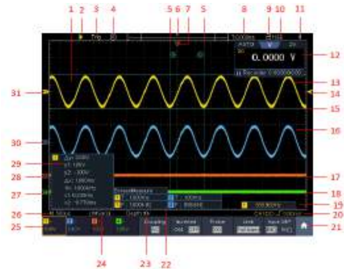
Рисунок 2-5 Интерфейс дисплея
