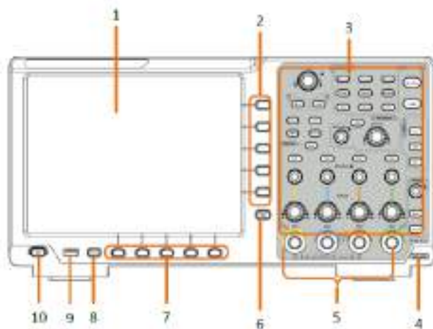
Рисунок 2-1 Передняя панель
